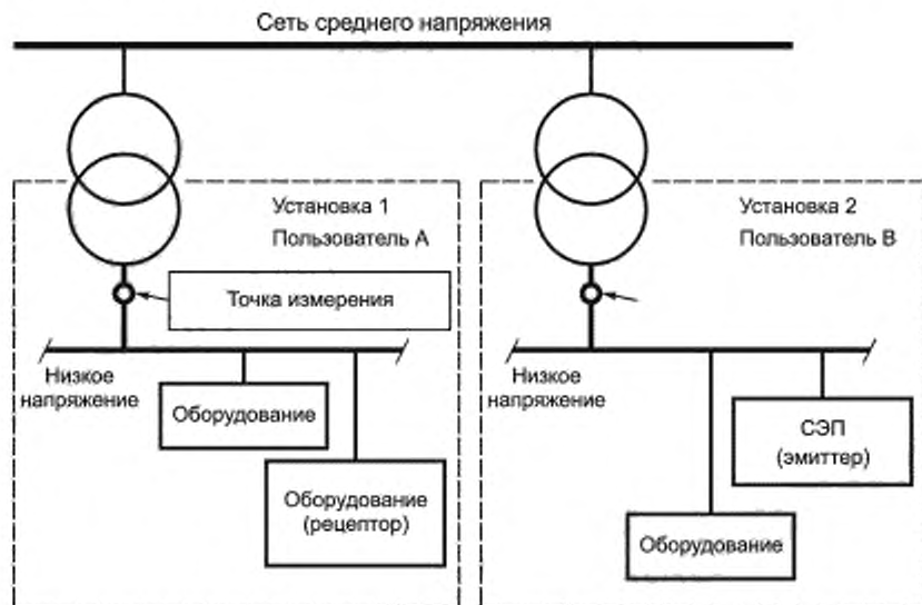
Рисунок 5 — Распространение помех
