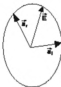
Рисунок D.3 — Вектор поляризации
