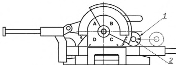
1 — фланец щупа; 2 — испытательный участок щупа
