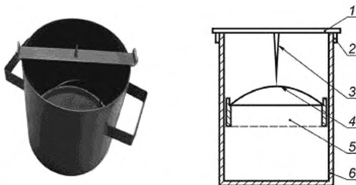
1 — металлическая пластина; 2 — ограничители; 3 — стрелка; 4 — петля; 5 — погружающий пуансон; 6 — цилиндрический сосуд
