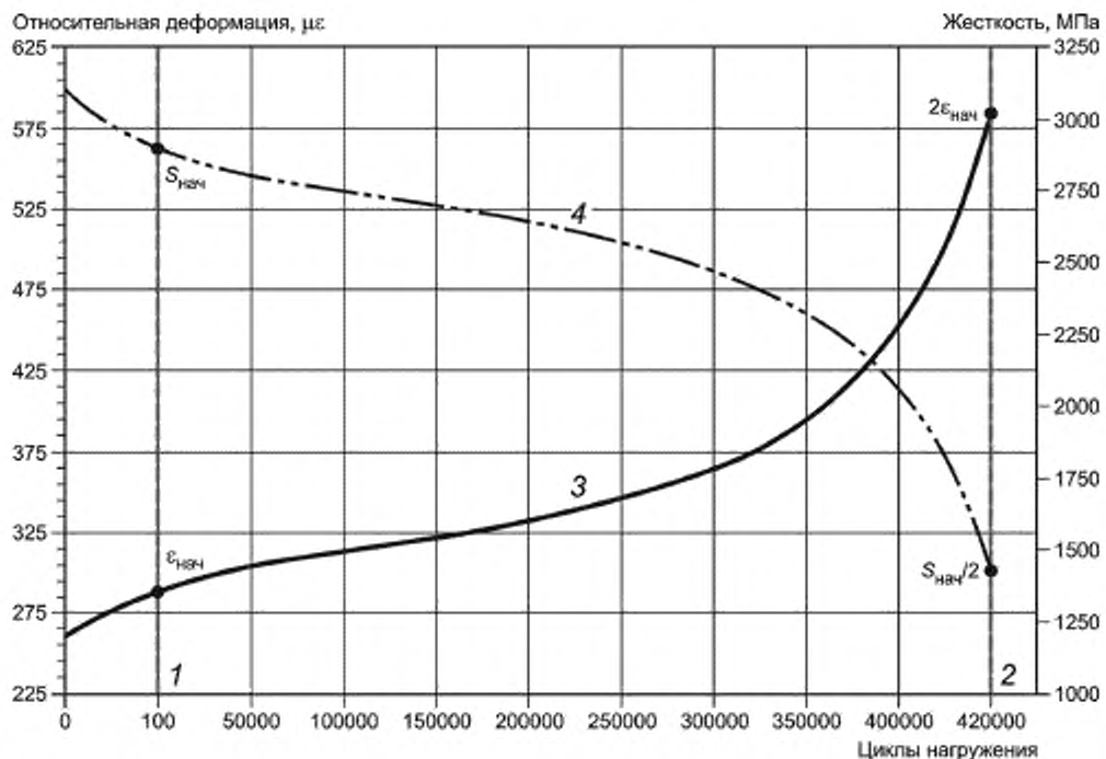
Рисунок 4 — Типовая зависимость относительной деформации и жесткости от количества циклов нагружения при испытании на усталостную долговечность
