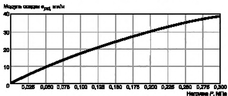
Рисунок А.3 — Компрессионная кривая пластичной пылеватой супеси
