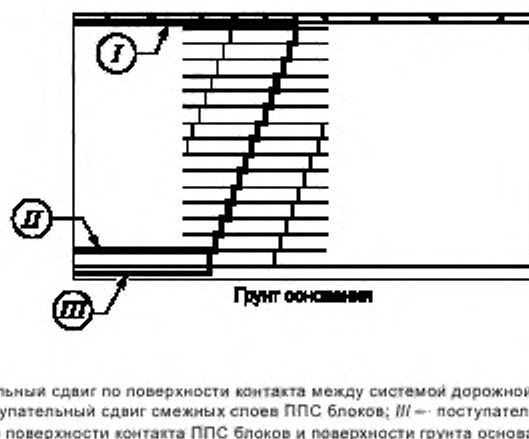
Рисунок 13 — Типовое поперечное сечение насыпи с вертикальными откосами с учетом трех видов разрушения
