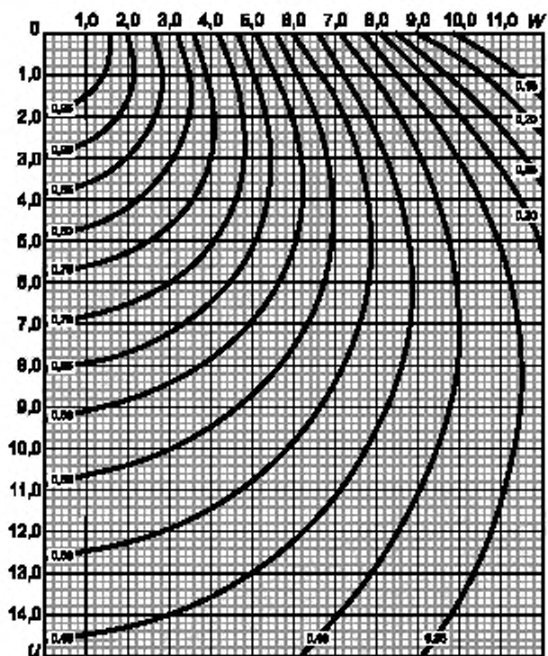
Рисунок В.12 — Графики значений при a_1 = \frac{\sigma_1}{\rho_0} \frac{2a}{B} = 10
