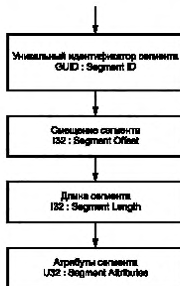
Рисунок 5 — Данные записи содержания файла
