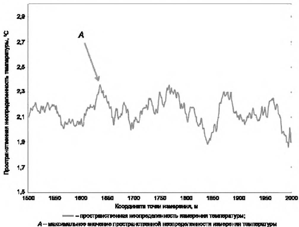
Рисунок 8 — Пример термограммы для определения пространственной неопределенности измерения температуры
