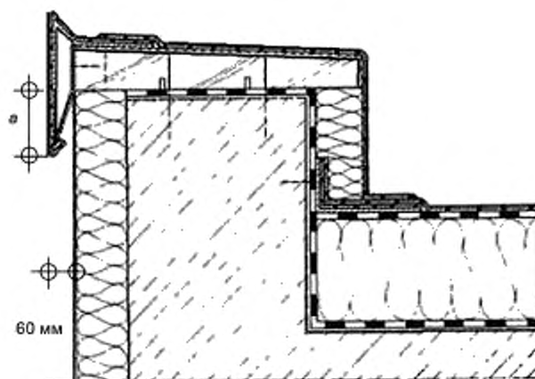
Рисунок 13 — Установка отлива по внешнему краю парапета
