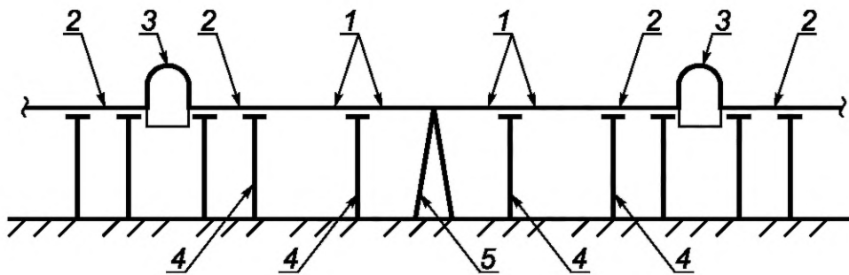
1 — средний пролет; 2 — крайний пролет; 3 — компенсатор; 4 — подвижная опора; 5 — неподвижная опора
