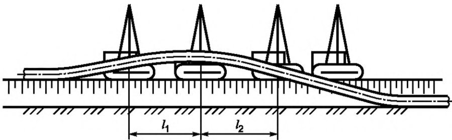
Рисунок А.2 — Схема расстановки трубоукладчиков при непрерывной укладке плети газопровода свыше DN\ 700 до DN\ 900 включительно
