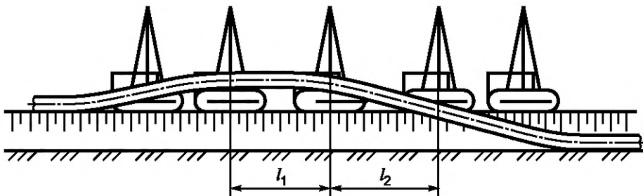
Рисунок А.4 — Схема расстановки трубоукладчиков при непрерывной укладке плети газопровода свыше DN\ 1200
