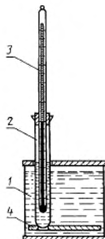
1 — масляная баня; 2 — стеклянная пробирка; 3 — термометр; 4 — металлический диск
