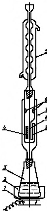
1 — электролитка; 2 — песочная баня; 3 — колба с n -гептаном; 4 — патрон с полимером; 5 — шариковый холодильник; 6 — отверстия; 7 — экстрактор; 8 — ловушка экстрактора; 9 — сифон
