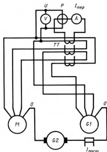
M — испытуемый двигатель; G1 — источник питания переменного тока; G2 — источник питания постоянного тока; 0, 0' — нулевые выводы обмотки; TT — трансформатор тока
