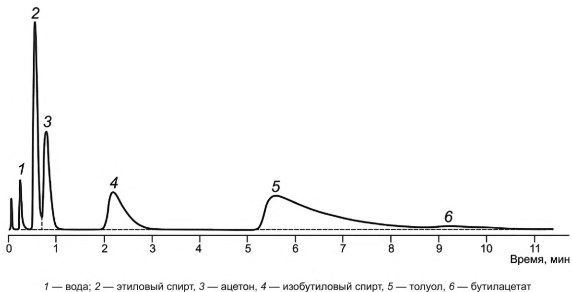
Рисунок Б.2 — Типовая хроматограмма растворителя марки 646
