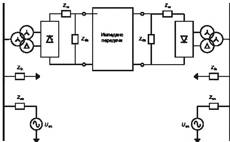
U_{\text{он}} — напряжение в системе переменного тока; Z_{\text{sn}} — сопротивление для гармоник в сети переменного тока; Z_{\text{fn}} — фильтры гармоник переменного тока; Z_m — сглаживающий реактор постоянного тока; Z_{\text{дн}} — фильтры постоянного тока
