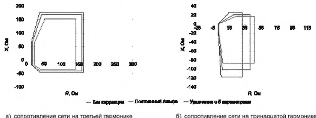
Рисунок Б.9 — Сопротивление сети для подстанции Aragaçuaга
