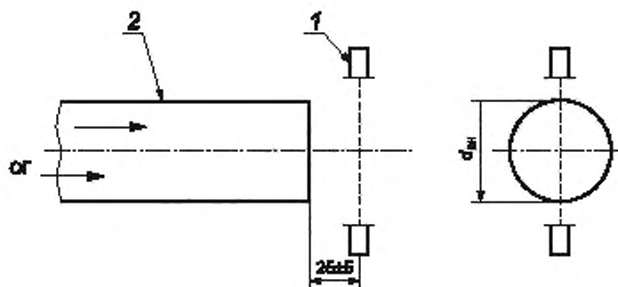
1 — полнооточный дыномер; 2 — выпускная труба круглого сечения, ОГ — поток ОГ; d_{вн} — внутренний диаметр выпускной трубы ( d_{вн} может быть приравнен к наружному диаметру выпускной трубы при толщине стенок менее 1,5 мм)
