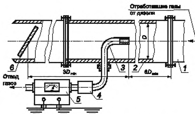
1 — выпускной трубопровод дизеля; 2 — выпускная труба испытательного стенда; 3 — газоотборник дыномера; 4 — ресивер; 5 — измерительный прибор; 6 — регулирующая заслонка
