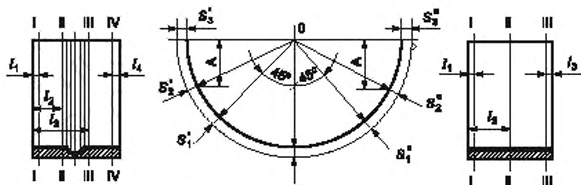
а) Вкладыши с кольцевой масляной канавкой
