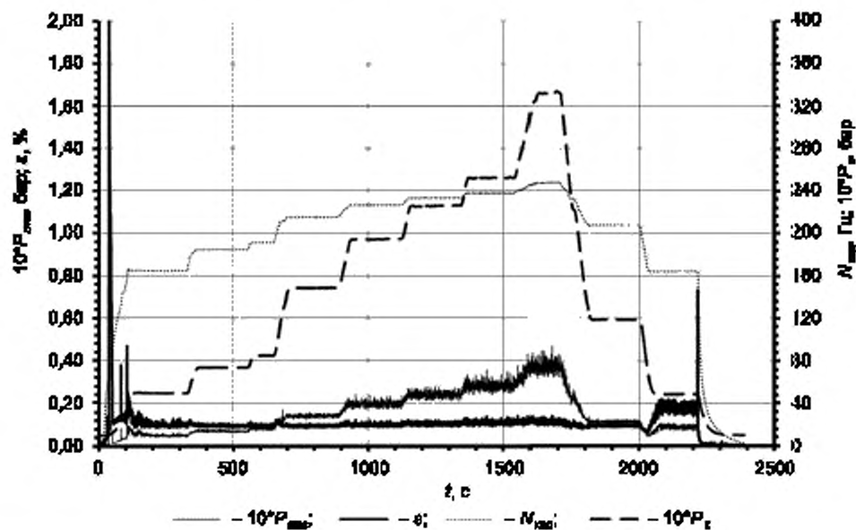
Рисунок Е.1 — Изменение частоты вращения КВД ( N_{вход} ), полного давления воздуха на входе в КС ( 10P_{ска} ), относительного ( \epsilon = P_{rms}/P_{\epsilon}^* ) и среднеквадратичного значения ( 10P_{rms} ) колебаний давления газа в зависимости от времени выхода газогенератора на заданные режимы работы
