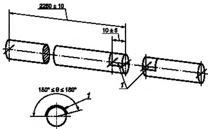
Рисунок 4 — Испытание сдвига оплетки, нарезка образца до заданной длины
