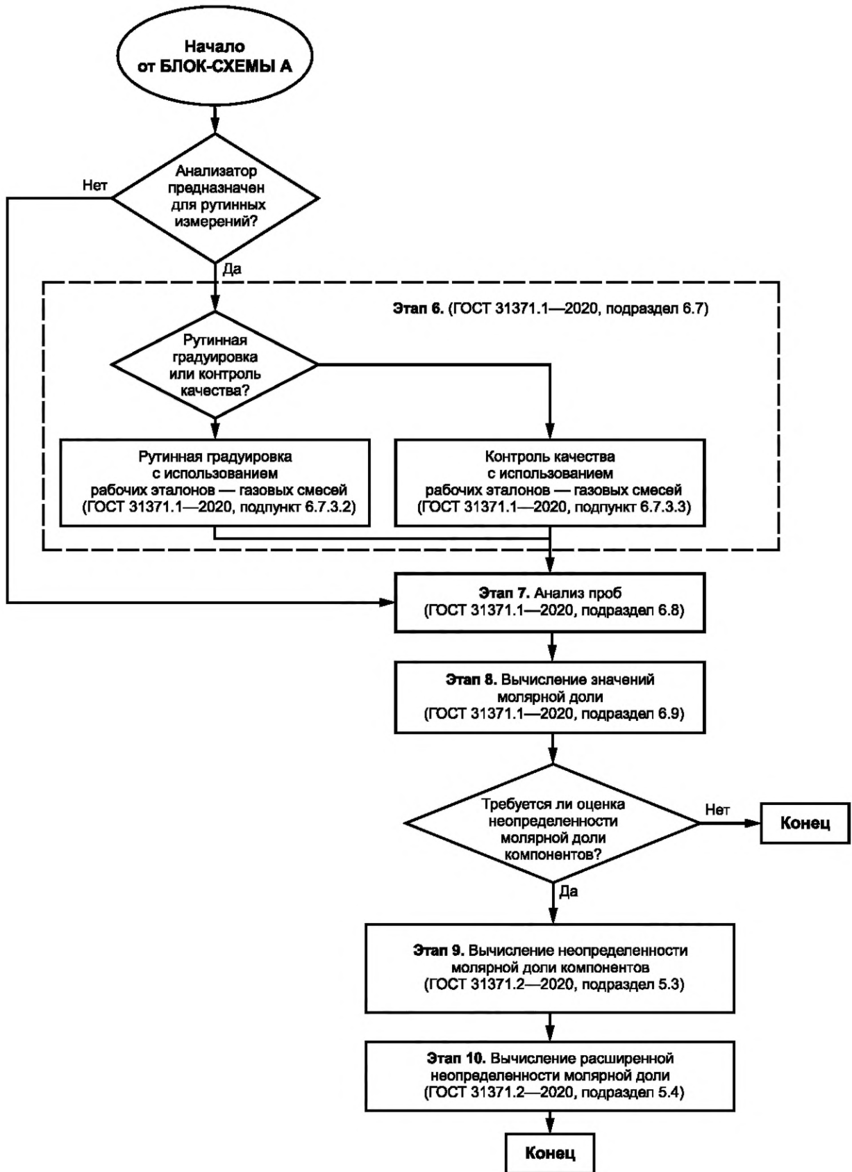
Рисунок 2 — Процедура определения молярной доли и неопределенности — этапы 6—10 (блок-схема В)
