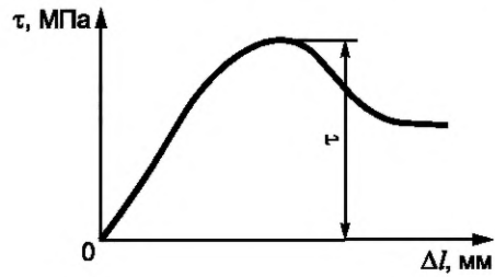
Рисунок А.1 — График \tau = f(\Delta l)
