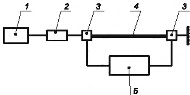
1 — оборудование растяжения; 2 — датчик растягивающего усилия; 3 — натяжная арматура крепления ОК; 4 — участок ОК, подвергаемый растяжению; 5 — средства измерений ОК; 6 — арматура крепления ОК
