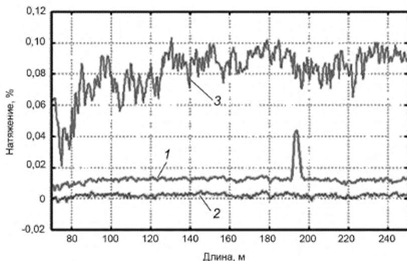
1 — ОВ имеет незначительное локальное натяжение; 2 — ОВ без натяжения; 3 — ОВ неоднородно натянута по длине кабеля, деформация значительная
