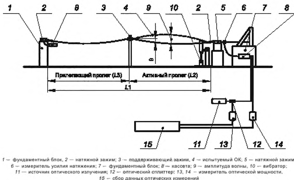
Рисунок 10 — Схема испытания ОК на воздействие галопирования
