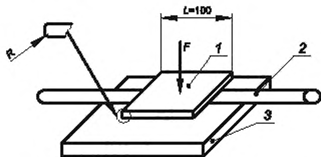
R , равный 5 мм, — радиус скругления кромок подвижной плиты; F — усилие, прикладываемое к подвижной плите в соответствии с документацией на ОК; L — длина плиты, l — перемещаемая плита, 2 — испытываемый образец ОК, 3 — неподвижная плита
