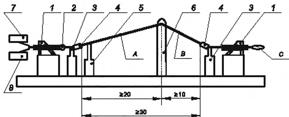
1 — концевой фундаментальный блок; 2 — датчик усилия натяжения; 3 — промежуточный фундаментальный блок; 4 — натяжной зажим; 5 — возбудитель колебаний; 6 — узел подвески; 7 — начало ОБ; 8 — конец ОБ; А — активный пролет; В — последующий пролет; С — соединение ОБ
