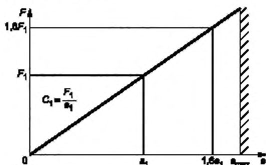
Рисунок 1 — Силовые характеристики пружинных комплектов ступени РП без упругого упора ( K_{\text{кз}} > 1,6 )
