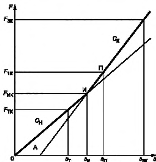
Рисунок 4 — Билинейная силовая характеристика пружинного комплекта
