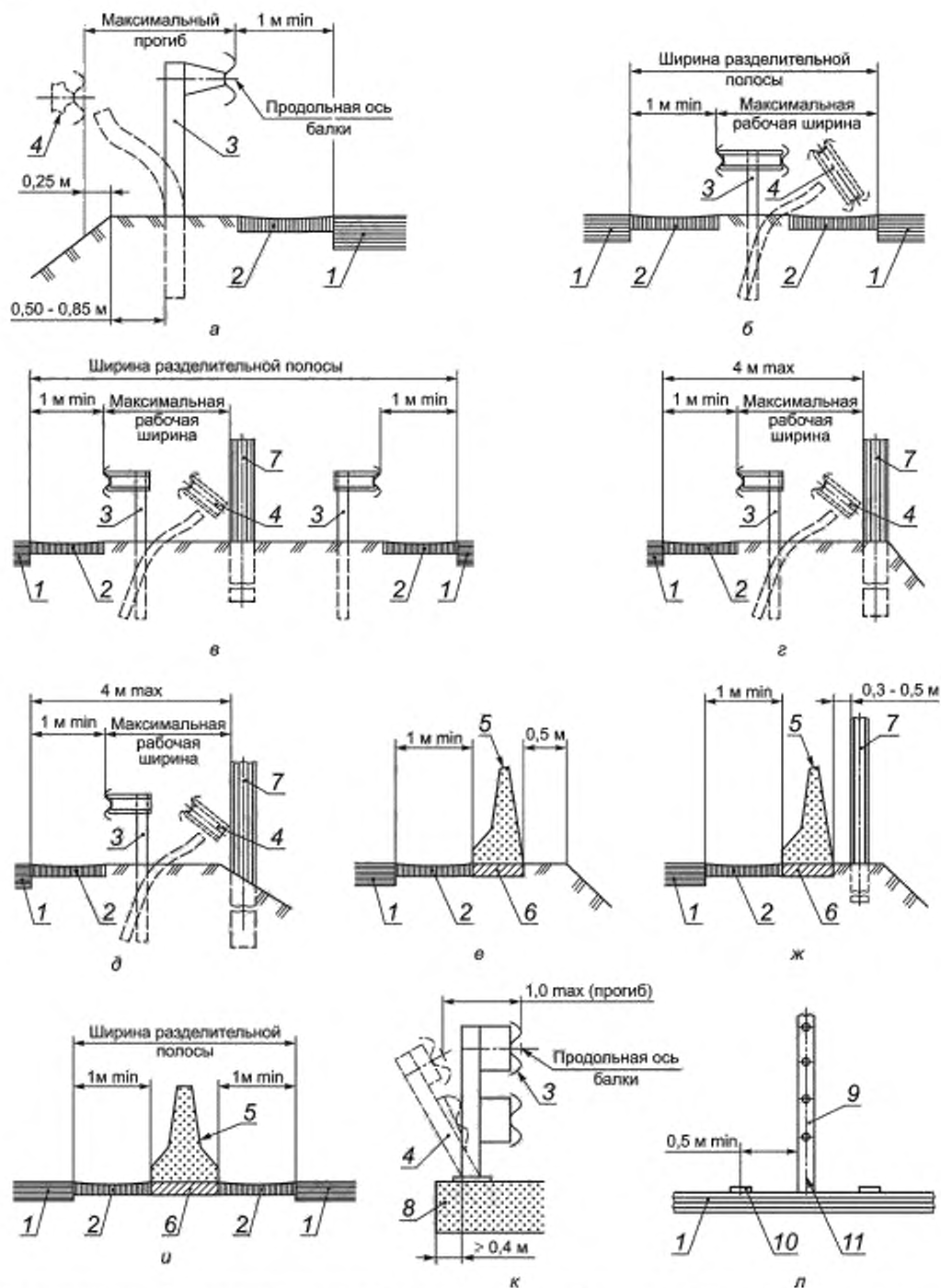
Рисунок В.28 — Примеры установки дорожных ограждений
