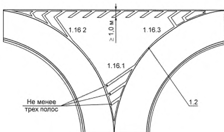
Рисунок В.12 — Пример нанесения разметки 1.16.1—1.16.3
