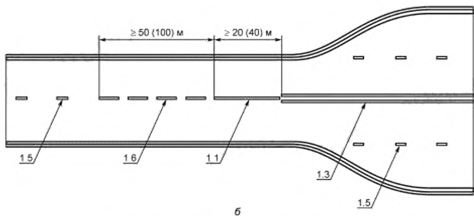
Рисунок В.8 — Пример нанесения разметки при уменьшении и увеличении количества полос для движения в одном направлении
