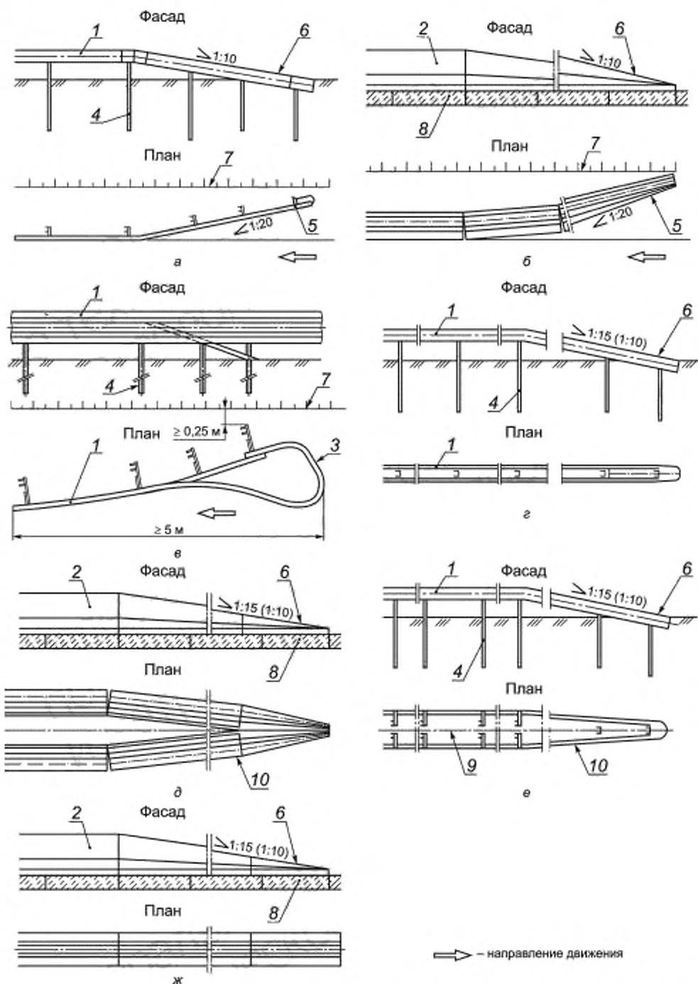
1 -- барьерное ограждение; 2 -- параллельное ограждение; 3 -- изгиб балки ограждения; 4 -- стойка ограждения; 5 -- отгон ограждения; 6 -- понижение ограждения на начальном и конечном участках; 7 -- бровка земляного полотна; 8 -- основание; 9 -- ось разделительной полосы; 10 -- сближение рядов ограждения с осью разделительной полосы
