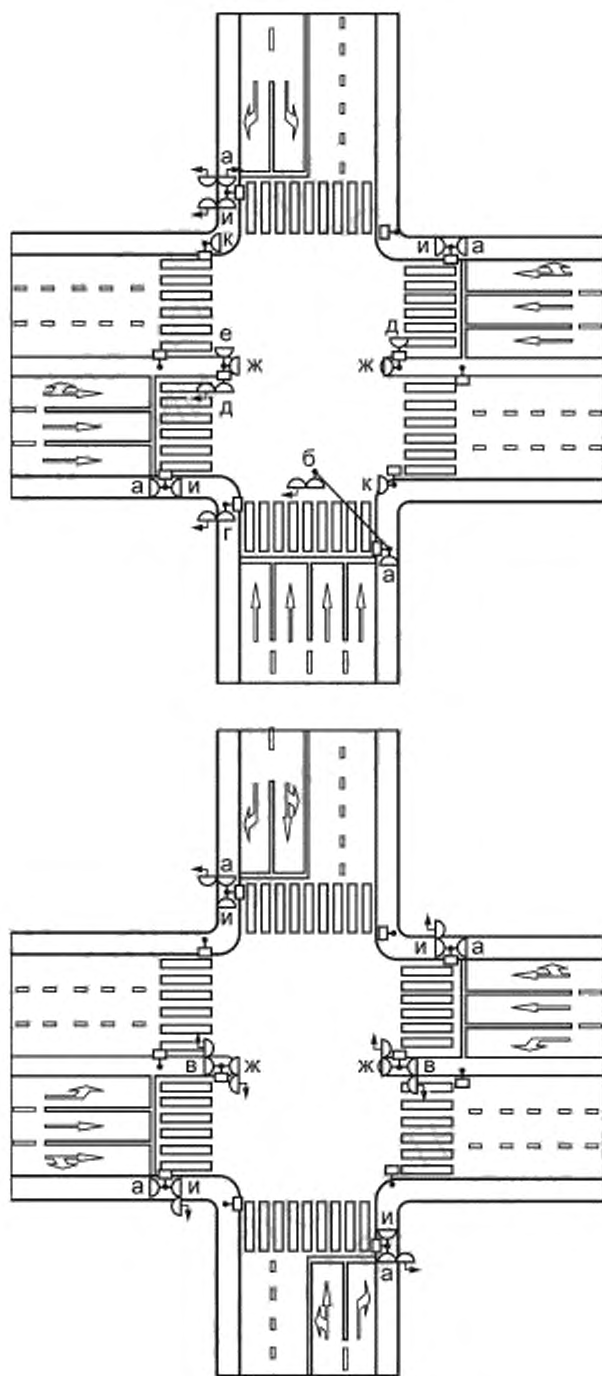
Рисунок В.26 — Места установки светофоров
