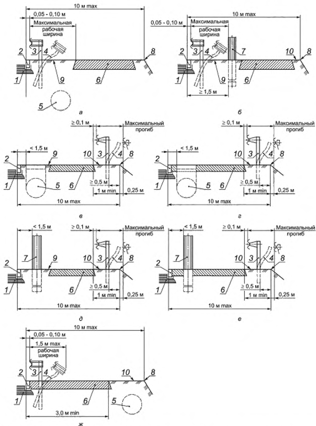
Рисунок В.29 — Примеры установки дорожных ограждений
