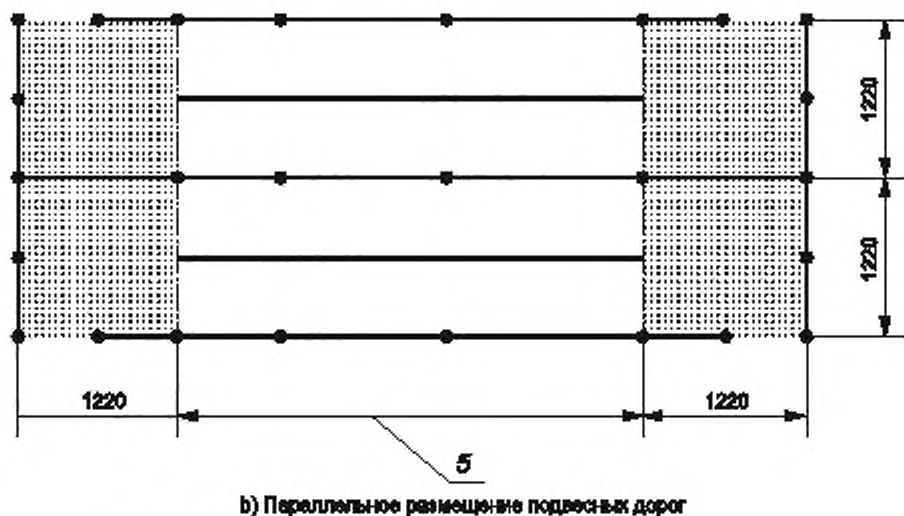
Рисунок 4 — Подвешенные дорожки — типовые схемы
