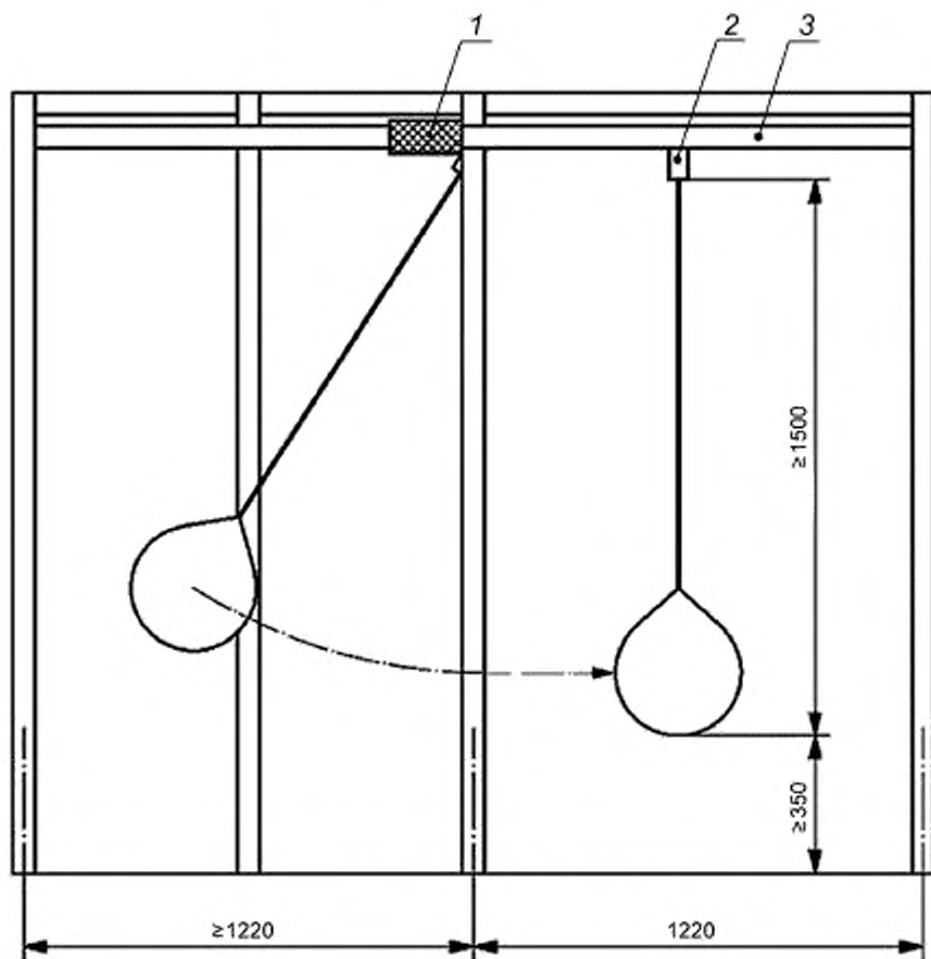
1 — сиденье; 2 — каретка; 3 — направляющая подвесной дороги
