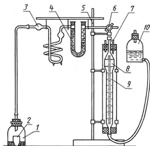
1 — реакционная склянка; 2 — фарфоровый тигель; 3 — спиральный прибор; 4 — U-образная трубка; 5 — металлический штатив; 6 — трехходовой кран; 7 — ртутный термометр; 8 — газоизмерительная бюретка; 9 — цилиндр; 10 — уравнительная склянка
