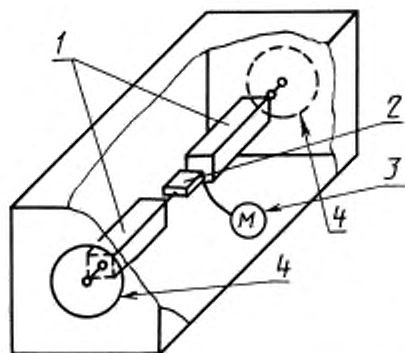
1 — сбалансированные безындуктивные сопротивления; 2 — термопара; 3 — индикаторное устройство; 4 — металлические пластины диаметром (170 ± 10) мм
