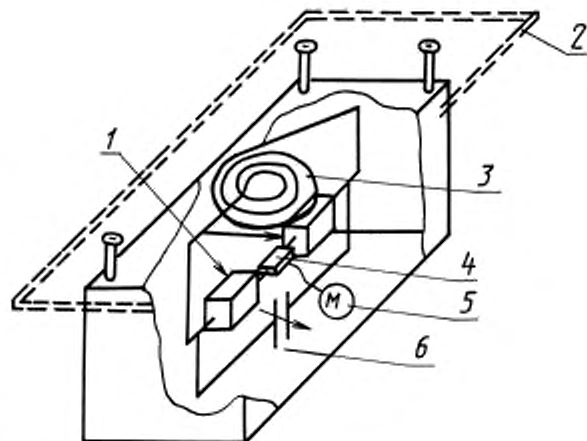
1 — сбалансированные безындуктивные сопротивления; 2 — изолирующая опорная плита с малыми потерями для испытываемых индукторов; 3 — катушка индуктивности; 4 — термопара; 5 — индикаторное устройство; 6 — конденсатор
