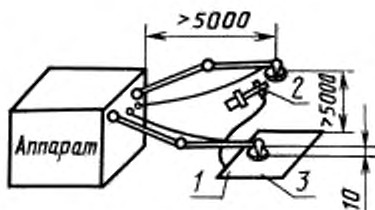
Испытание электрической прочности на высокой частоте (см. 20.2)
