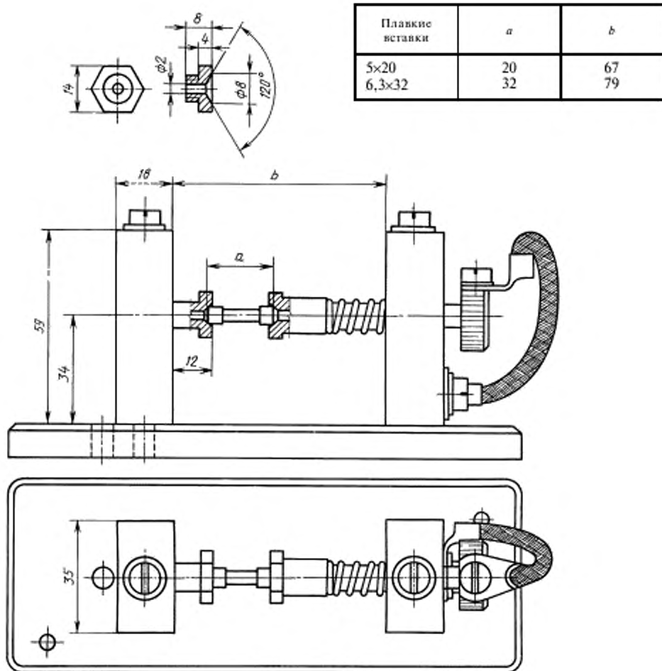
Рисунок 3 — Цоколь для испытаний на отключающую способность (см. 4.3.1)
