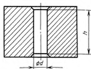
Рисунок 4 — Калибр для проверки на соосность (см. 5.4)
