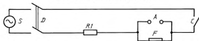
Рисунок 6 — Типовая схема для испытаний на отключающую способность плавких вставок с низкой отключающей способностью (см. 6.3)
