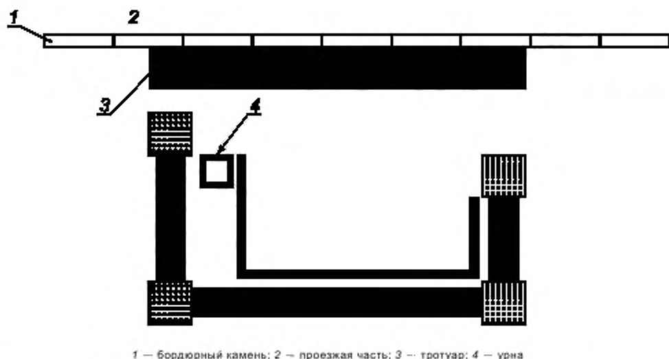
Рисунок А.8 — Применение ТНУ для обустройства тактильно обозначенных путей следования вдоль стен остановочного павильона и поля посадки в маршрутные транспортные средства
