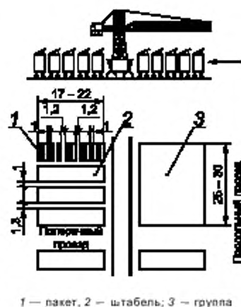
Рисунок А.5 — Планировка групп штабелей при укладывании башенным краном пиломатериалов рассеянно-сосудистых пород, кроме граба и клена
