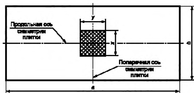
a , b — длина и ширина плитки, x , y — длина и ширина вырезаемого образца
