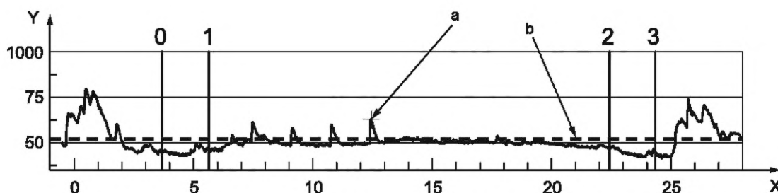
Y — уровень звука с частотной коррекцией по шкале А, дБА; X — время, с; а — максимальный уровень звука; b — эквивалентный уровень звука L_{Aeq}
