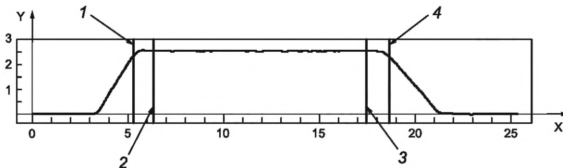
Y — скорость, м/с; X — время, с; 1 — 95 % максимальной скорости на участке ускорения; 2 — 1 с после 95 % максимальной скорости на участке ускорения; 3 — 1 с перед 95 % максимальной скорости на участке замедления; 4 — 95 % максимальной скорости на участке замедления
