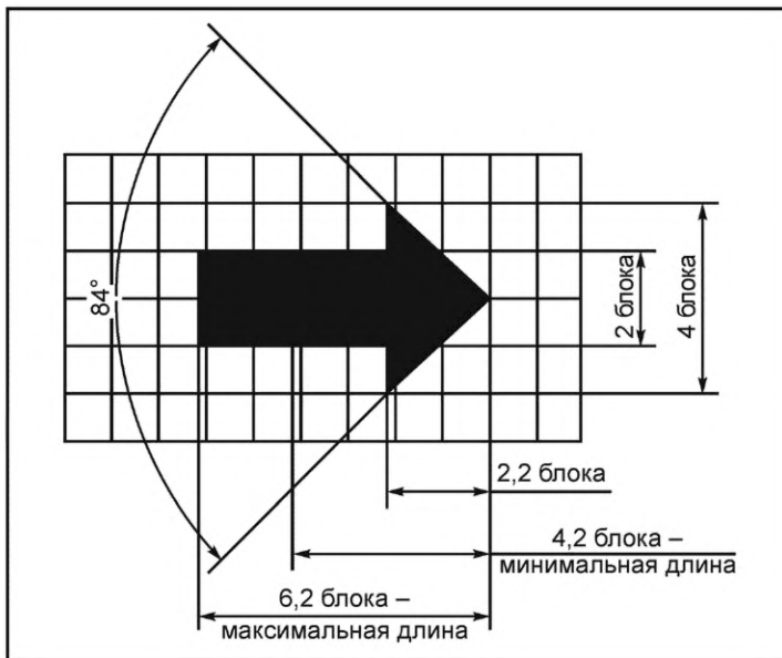
Рисунок Г.22 — Стрелка для отображения направления давления или усилия
