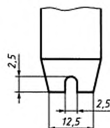
Рисунок 14 — Конечный вырубной нож с выемкой
