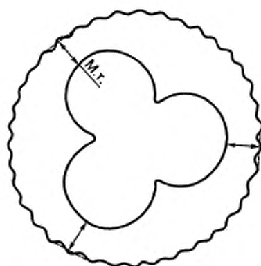
Рисунок 9 — Измерение толщины оболочки (наружная поверхность неправильной формы)
