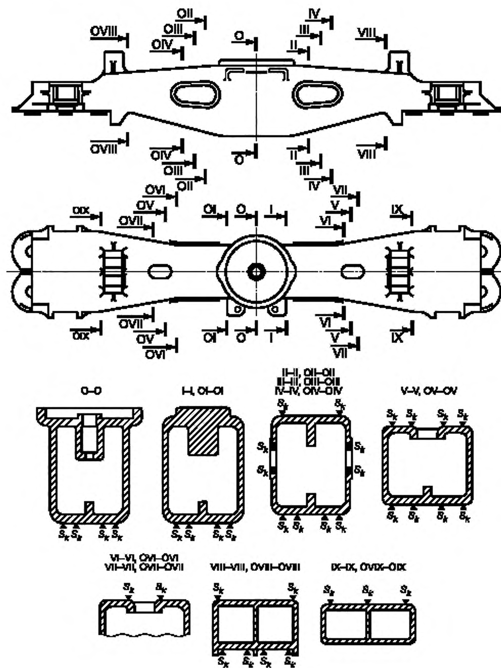
Рисунок 2 — Схема установки тензорезисторов для измерения напряжений и сил, действующих на надressорную балку
