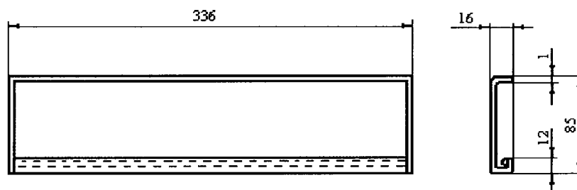
Рисунок 3 – Противень
