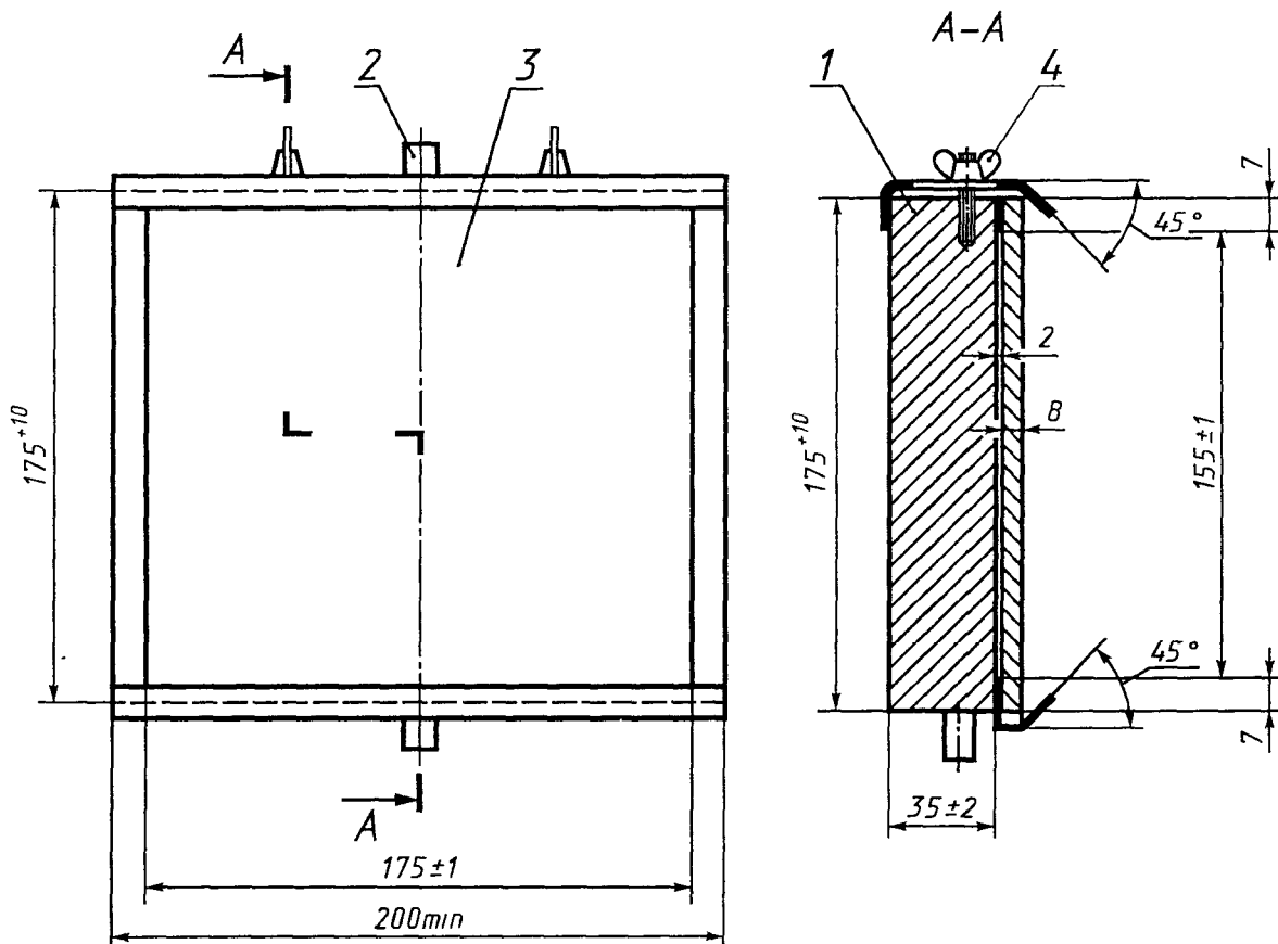
Рисунок 6 - Ударный элемент маятника для механических испытаний (см. 9.2.5.2.1)
