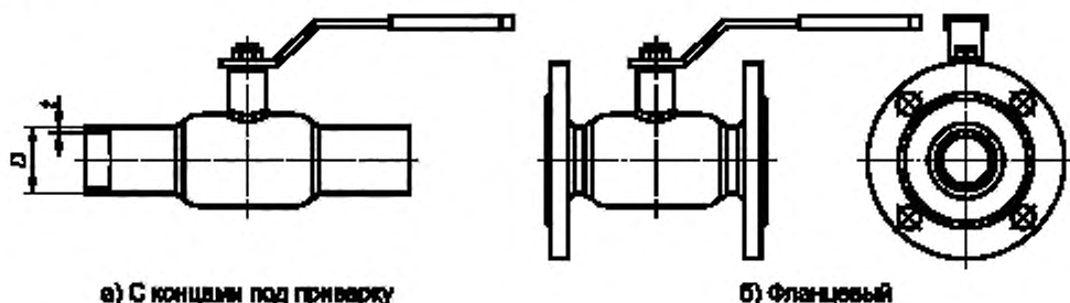
Рисунок 1 — Цельносварной шаровой кран с плавающей пробкой
