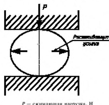
Рисунок 2 — Схема испытания на прочность при диаметральной разрыве
