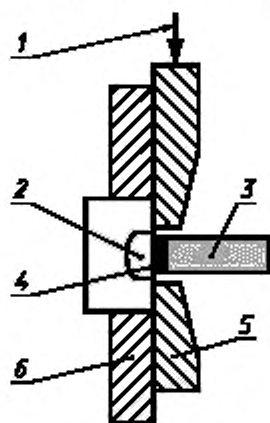
1 — нагрузка; 2 — субстрат — фрагмент зуба в монтировочной пластмассе с открытой для испытания поверхностью эмали; 3 — испытываемый восстановительный материал; 4 — адгезив; 5 — нагружающая пластина в приспособлении для сдвига; 6 — кольцо в приспособлении для сдвига
