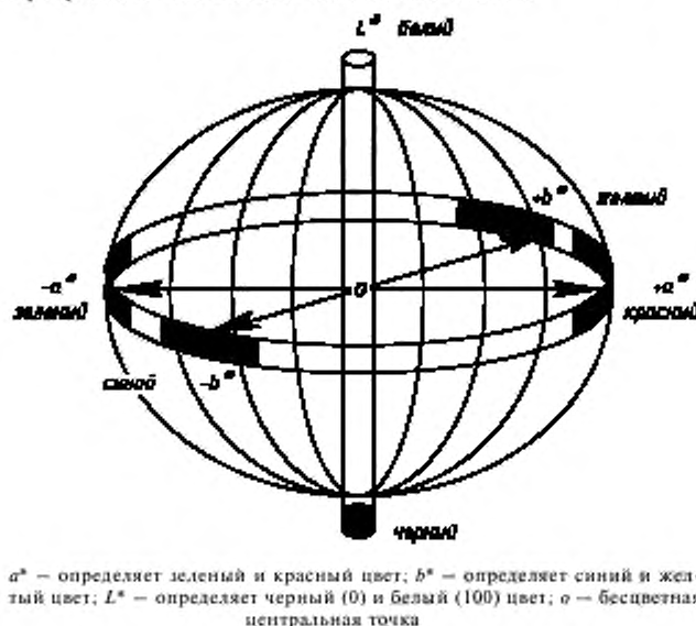
Рисунок 6 — Международная система CIELAB для аппаратного измерения цвета
