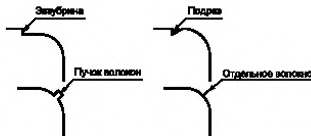
Рисунок 4а — Дефекты кромки, показанные на примере скругленного угла
