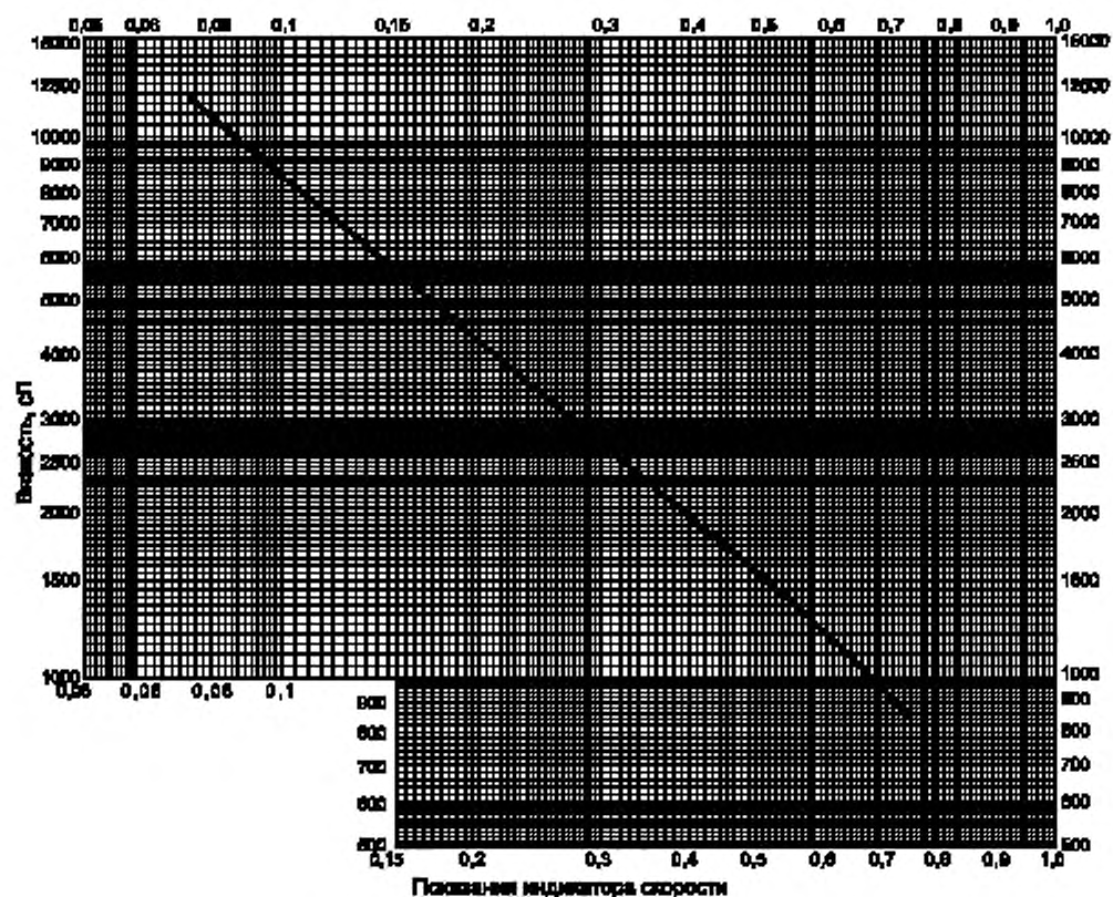
Рисунок 4 — Типичная диаграмма калибровки
