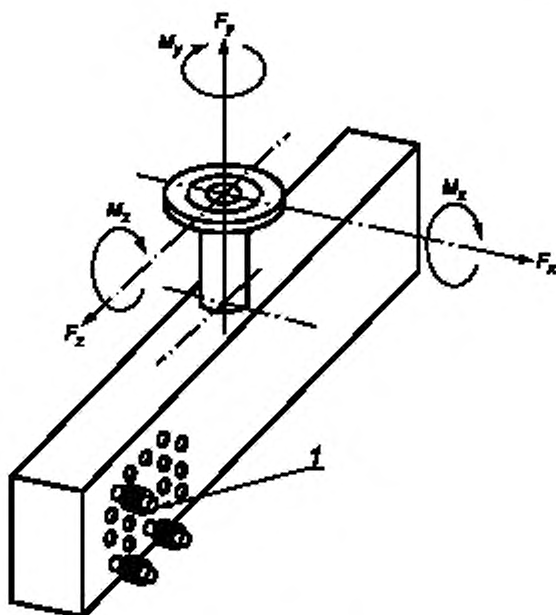
1 — оребренные трубы
