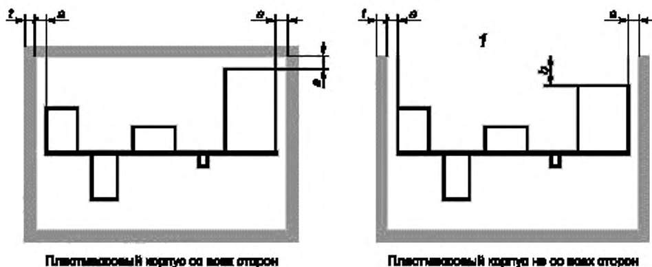
Рисунок 3 — Расстояния между стенкой или наружной поверхностью компаунда и элементами или проводниками
