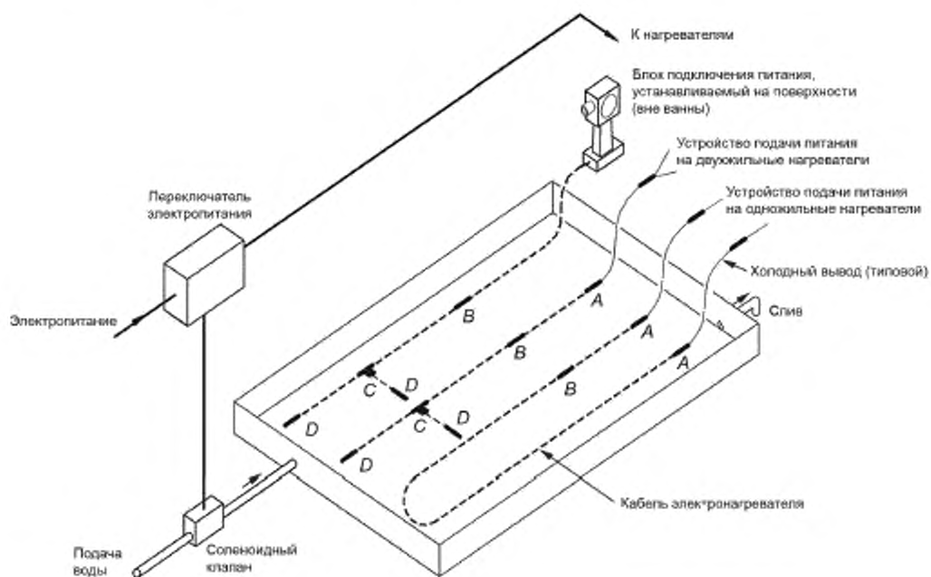
A — встроенный силовой соединитель, B — встроенный соединитель нагревательного элемента, C — встроенный T-образный соединитель; D — встроенный концевой соединитель
