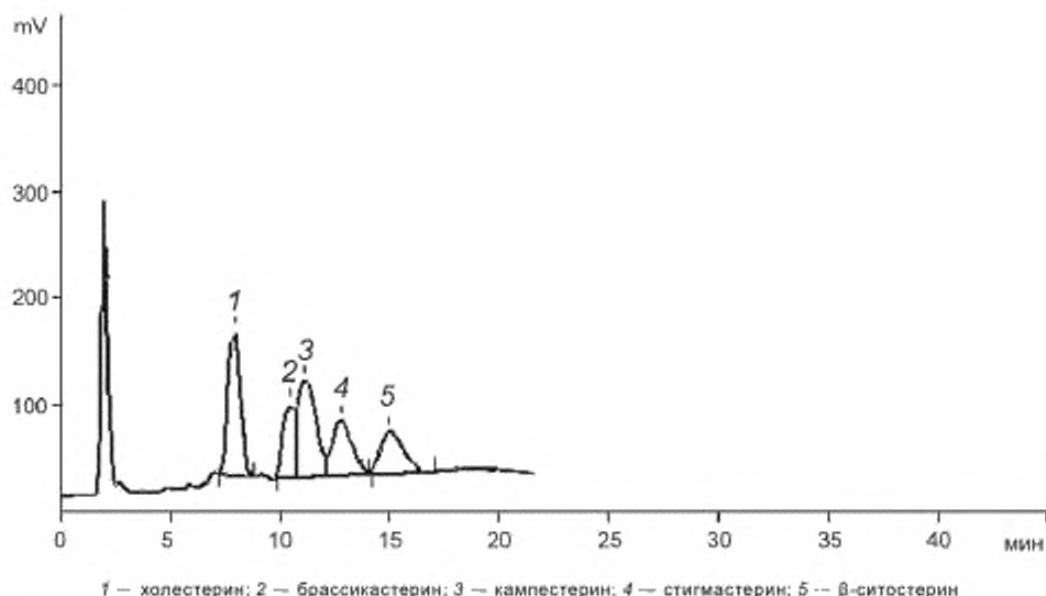
Рисунок 1 — Хроматограмма смеси стандартов стеринов
