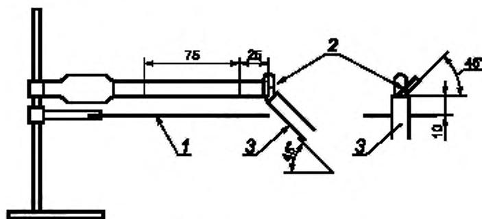
1 — металлическая сетка; 2 — образец; 3 — горелка
