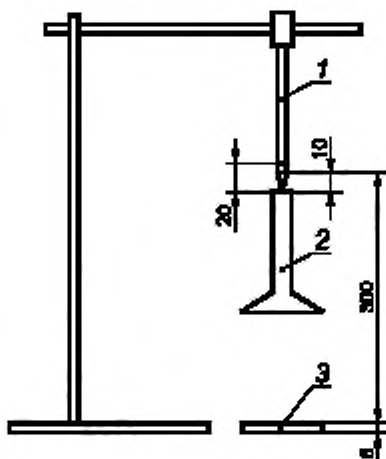
1 — образец, 2 — горелка; 3 — вата
