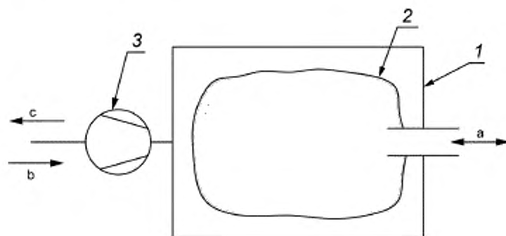
1 — емкость для проб; 2 — корпус емкости для проб; 3 — вентилятор; a — отбираемая или подаваемая проба воздуха, b — выпуск воздуха из емкости; c — заполнение воздуха емкости
