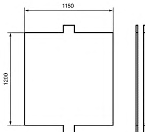
Рисунок С.2 — Емкость для проб в разрезе
