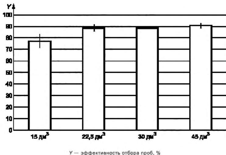
Рисунок 1 — Эффективность отбора проб для крупных спор ( Cladosporium ) при различных скоростях расхода воздуха
