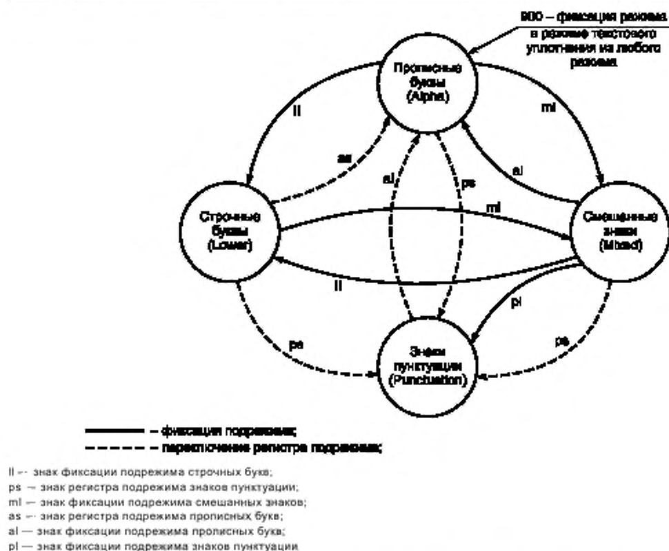
Рисунок 6 — Переключения подрежимов в режиме текстового уплотнения
