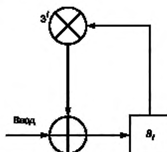
Рисунок К.1 — Делитель синдрома символа
