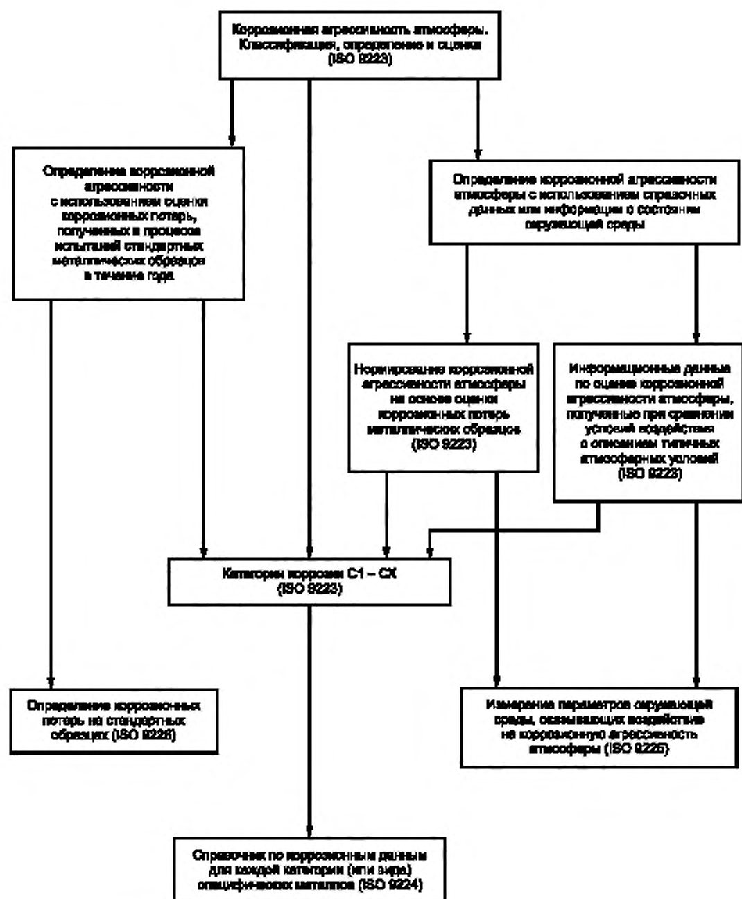
Рисунок 1 — Классификация атмосферной коррозии
