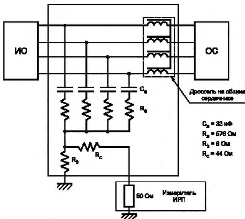
Рисунок В.4 — Эквивалент полного сопротивления сети для применения с двумя незранированными симметричными парами (вариант 2)
